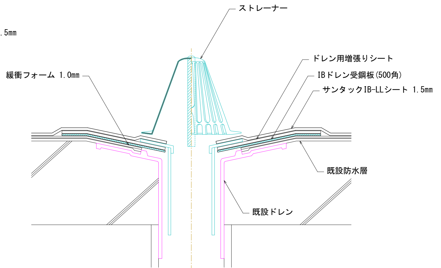
ドレン納まり図
