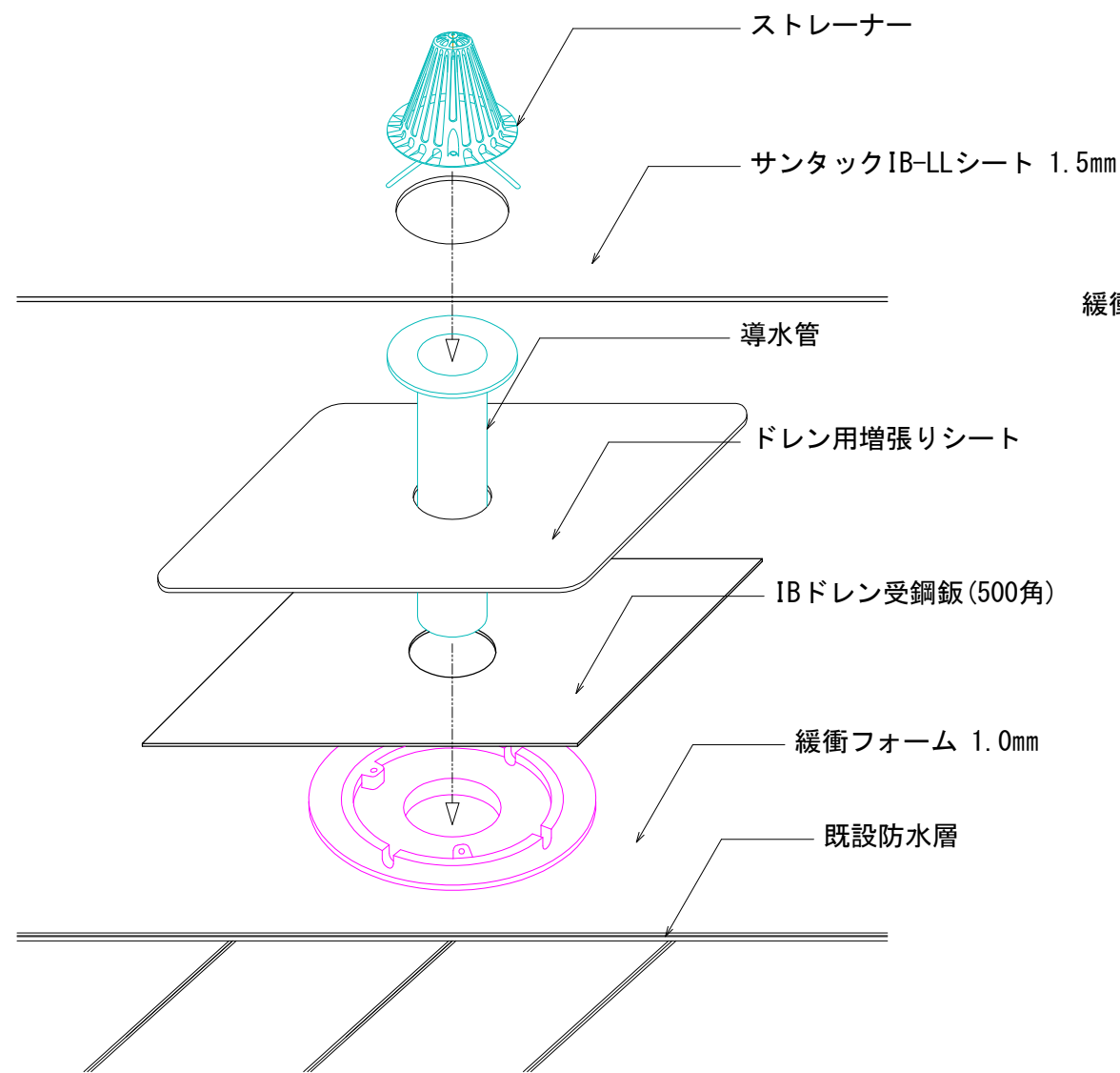
ドレン部納まり手順 S=1:8
